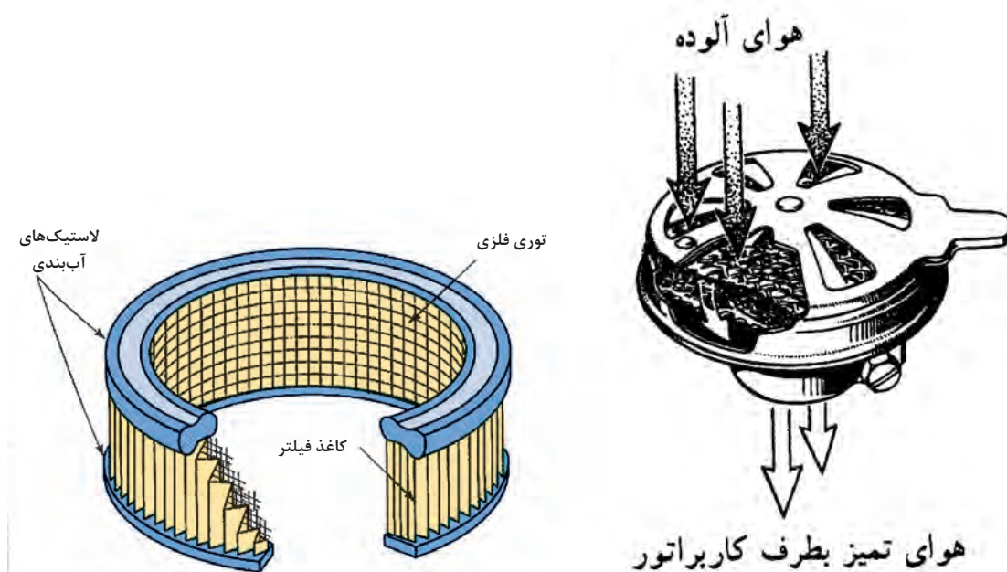
شکل ۱-۵۳ هواکش کاغذی
