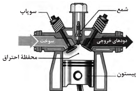
شکل ۵-۱- محفظه احتراق
