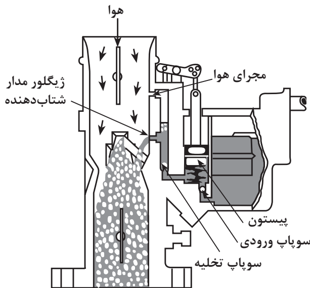
شکل ۱-۷۱ مدارهای کاربراتور
